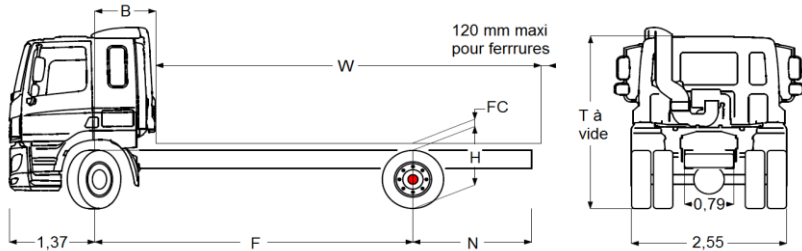
( FC ) Mini : 150 mm avec pneumatiques 315/70R22.5 et longerons 260 mm.
