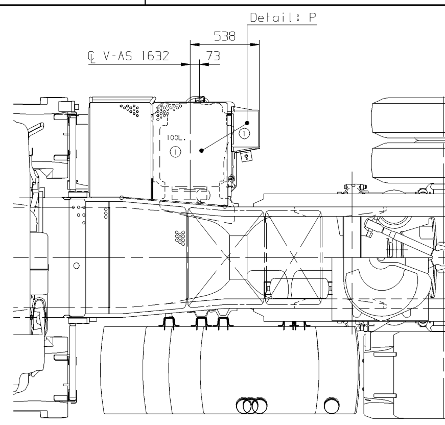
Situatie 100L. AdBluetank Version 100L. AdBluetank
