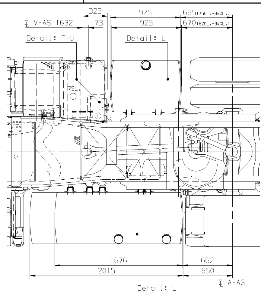
Situatie 620L./750L. + 340L. Version 620L./750L. + 340L.
