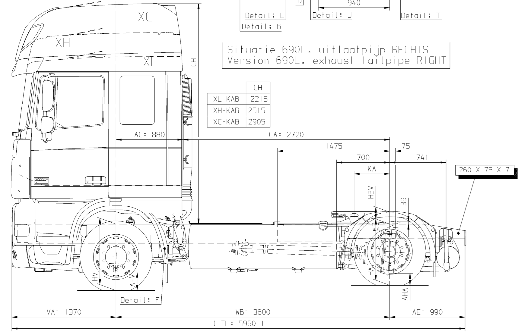
Getekende situatie XF105. Drawing represents XF105. Le plan se rapporte au XF105. Situation auf Zeichnung XF105. — LHD XC-cab.
