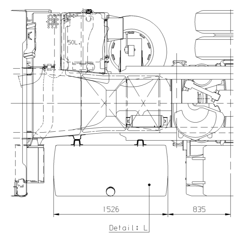
Situatie 525L. uitlaatpijp LINKS of RECHTS Version 525L. exhaust tailpipe LEFT or RIGHT
