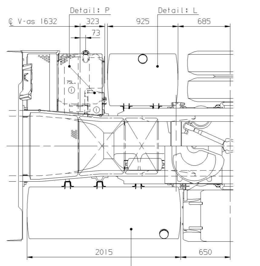
Situatie 750L. + 340L. Version 750L. + 340L.
